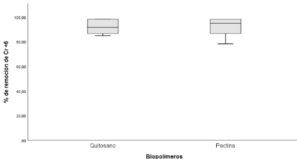
Figura 1. Distribución de datos de remoción de Cr +6 con pectina y quitosano.
