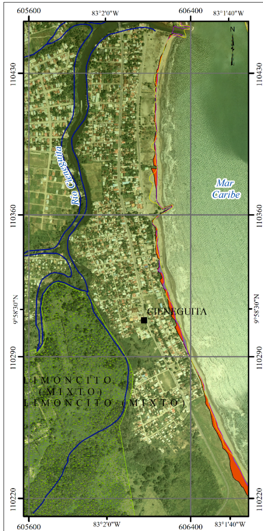
Figura 3.a. Puntos calientes Playa Cieneguita
