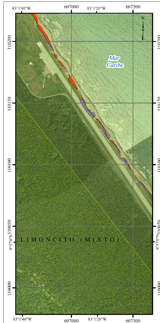
Figura 3.b. Puntos calientes Aeropuerto de Limón
