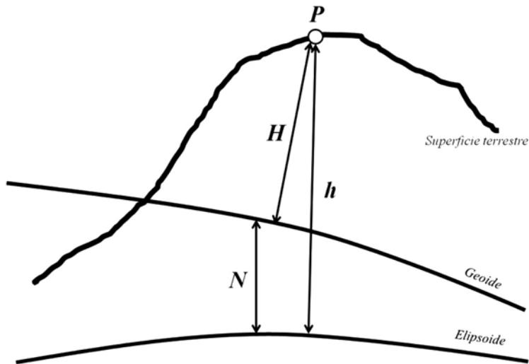
Figura 6. Relación entre la altura física referida al geoide, la altura elipsóidica referida al elipsoide y la ondulación del geoide
