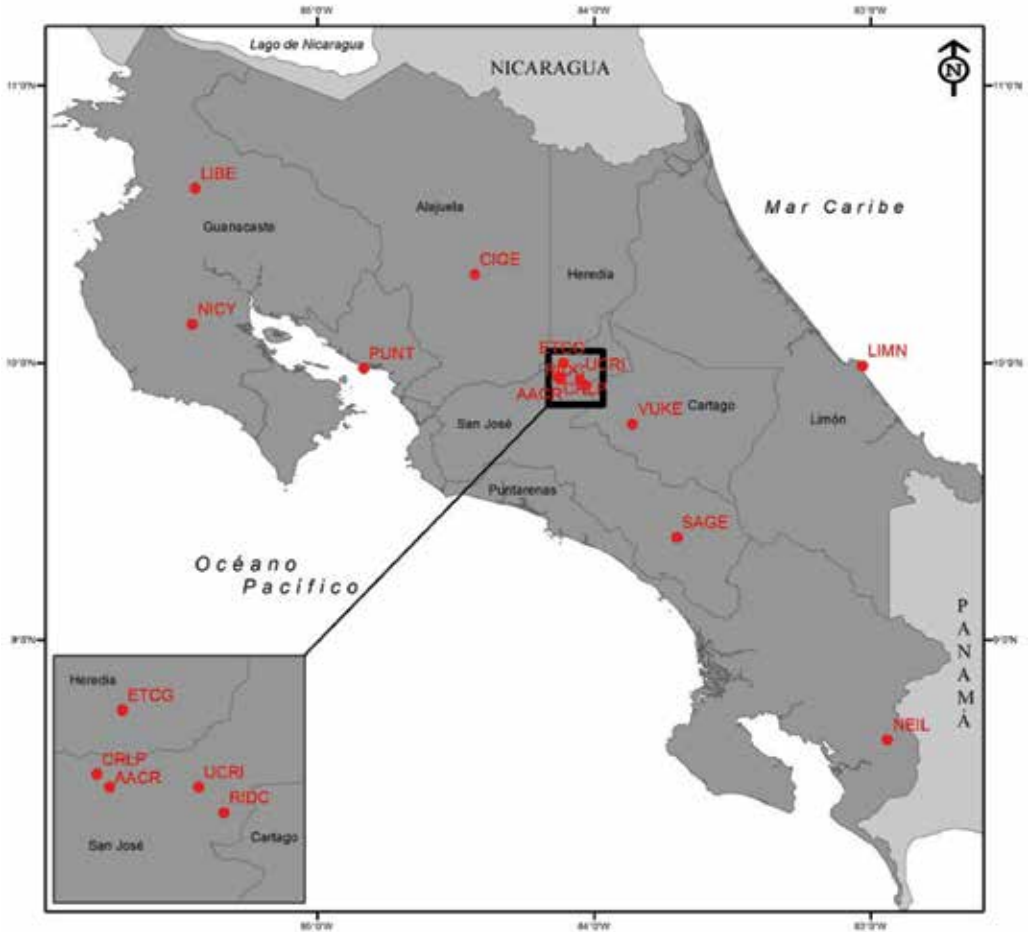
Figura 6. Ubicación de las estaciones GNSS de Costa Rica integradas a la red SIRGAS-CON
