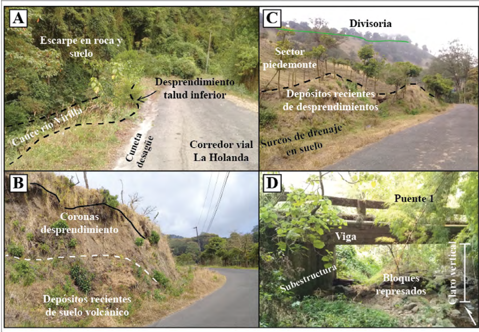
Figura 13. A), B) y C) Vista de desprendimientos recientes a lo largo del corredor vial La Holanda que atraviesa el área de estudio, notorio los escasos desagües pluviales. D) Claro vertical de 2,8 m en el Puente 1 y materiales represados.
