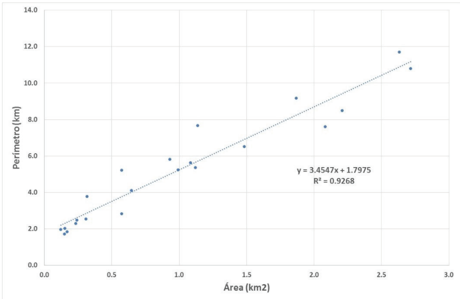
Figura 3. Correlación del área contra el perímetro de las 22 microcuencas, subcuenca del río Páez.
