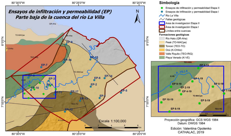
Figura 18. Localización de los ensayos de infiltración y permeabilidad en las Etapas I y II
