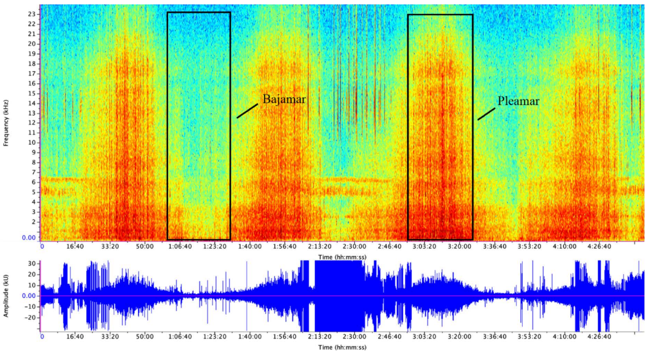
Fig. 2. Visualización de espectrograma y oscilograma correspondiente a dos días de grabaciones del sitio 3-Rompiente en Punta Morales. La escala de tiempo en la figura corresponde a la unión de audios de un minuto cada diez minutos durante aproximadamente 48 horas, por lo que no debe ser interpretada como una escala de tiempo continua
