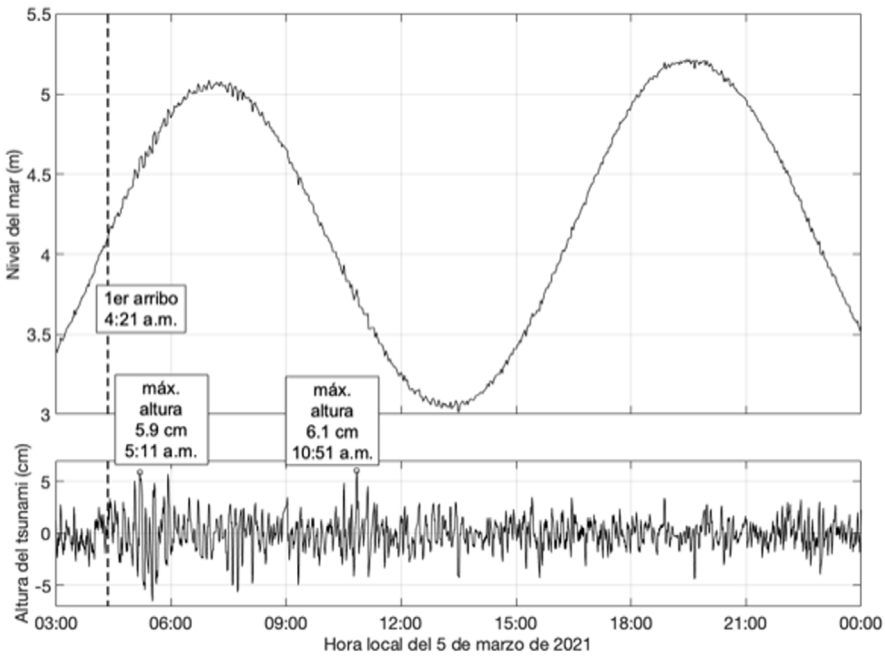
Fig. 4. Panel superior: mareograma original en la isla del Coco. Panel inferior: mareograma filtrado para mostrar únicamente el tsunami. El primer arribo fue a las 4:21 a. m. y la máxima altura sucedió a las 5:11 a. m. con un valor de 5.9 cm, mientras que el segundo ciclo de ondas obtuvo una altura máxima de 6.1 cm a las 10:51 a. m.
