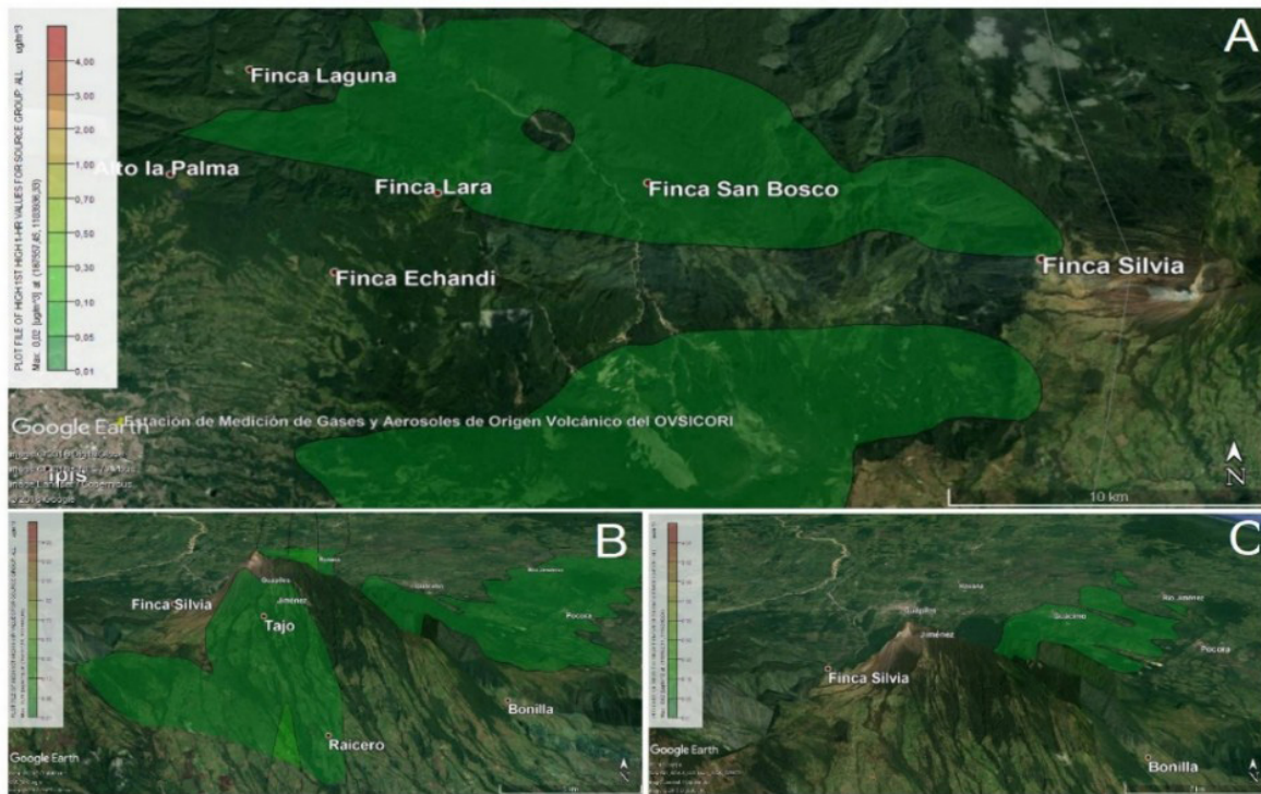
Figura 5. Modelos de dispersión de gases y partículas (AERMOD) del Laboratorio de Química de la Atmósfera (LAQAT-UNA) de los muestreos del 22/08/2018 (A), 05/10/2018 (C) y 05/04/2019 (B).
