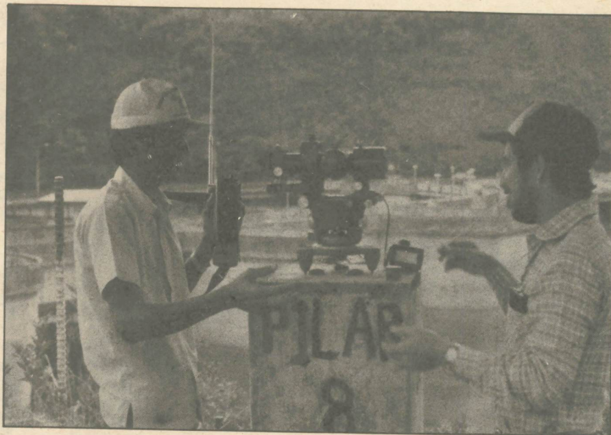
Estudiantes efectúan observaciones de ángulos desde un pilar que pertenece a la Red de Control Geodésico en la Represa de Cachí.
