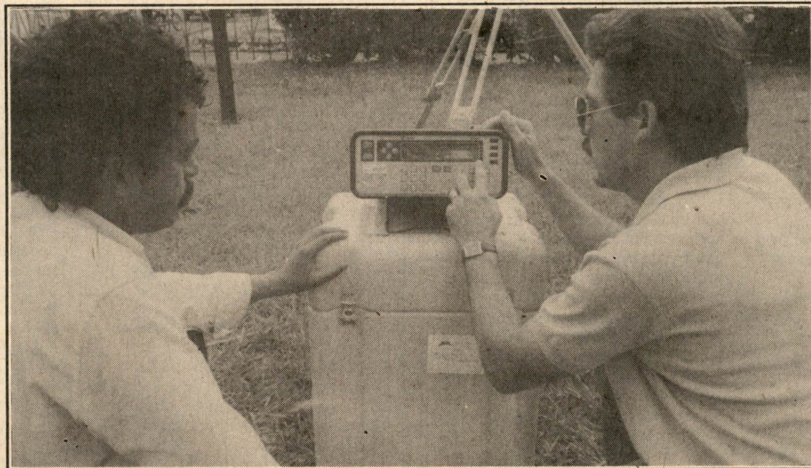
Los topógrafos Tomás Marino y Franklin De Ovaldía del OVSICORI prueban el receptor del satélite. Este equipo permite establecer coordenadas tridimensionales con gran exactitud y fue prestado por la NASA.
