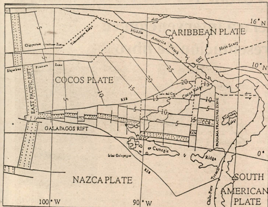
Distribución de la edad litosférica en millones de años de la Placa del Coco. El mapa base es un segmento del Mapa de Tectónica de Placas de la región Circum-Pacífica, cuadrante sureste.
